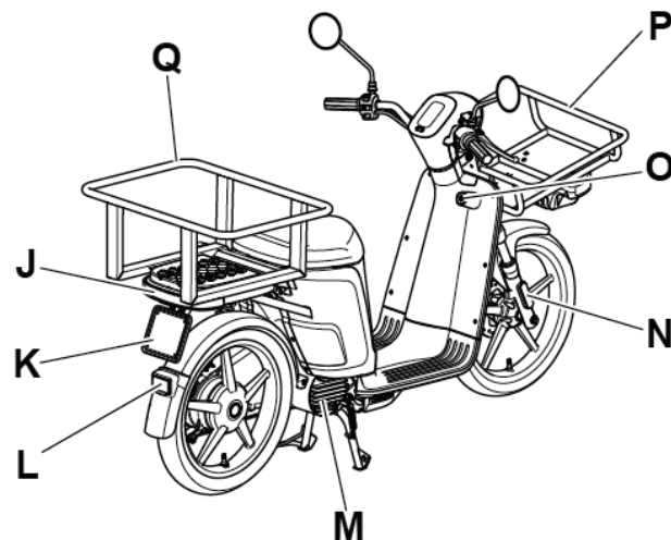
eSPRO 45K - eSPRO 70K right side
